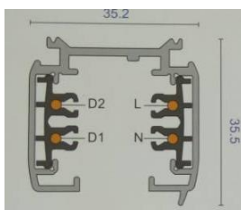
4 Wire DALI, vid standard 3-fas skena
