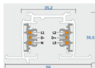
6 wire DALI, 3-fas eller så använder ni en 3-fas skena med 6 anslutningar och så använder vi en 3-fas DALI adapter för 6 anslutningar/wires till de linjära Track LED.
